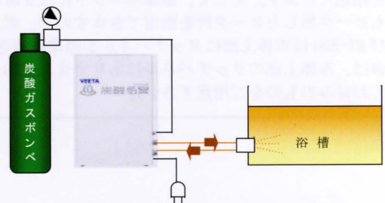
浴槽に循環金具を取り付ける場合
